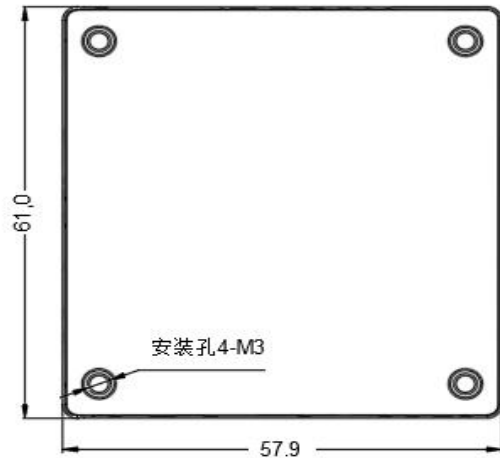
标准型 61.0*57.9*12.7mm
